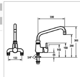
Kraangat - Perçage utile : Ø 30 mm
